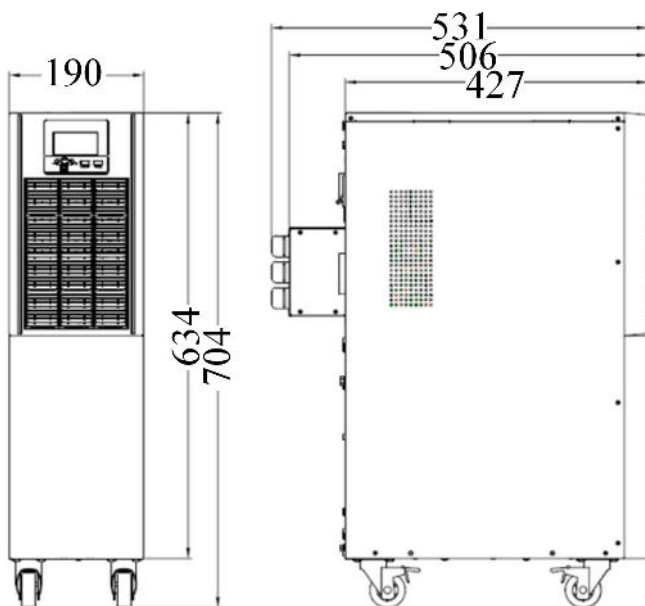
2. Modelos 4 a 8 kVA - Baterias internas (Padrão)
