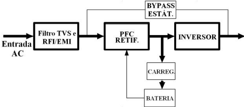
Fig 1- 4: Modo Normal
