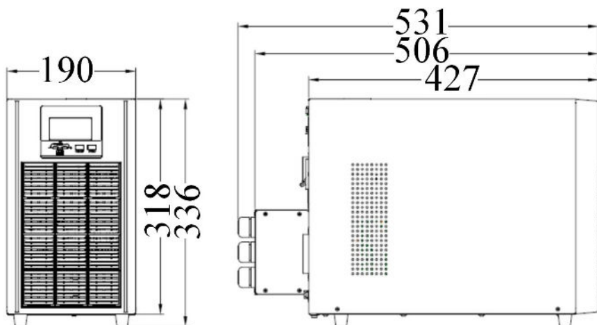
1. Modelos 4, 5, 6 e 8 kVA - Bateria externa (Long)
