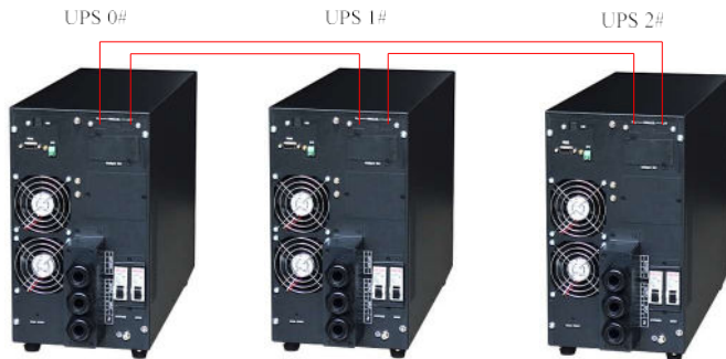
Fig 2- 4: Sistema Paralelo Nobreak
