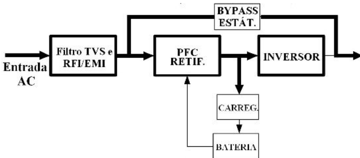
Fig 1- 7: Modo ECO
