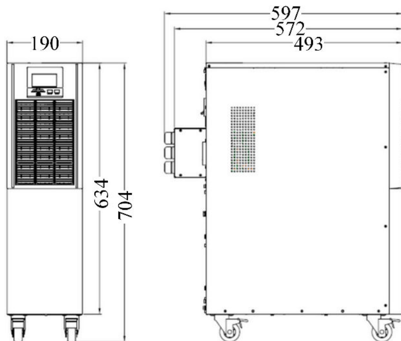
4. Modelos 10 e 12 kVA - Baterias internas (Padrão)
