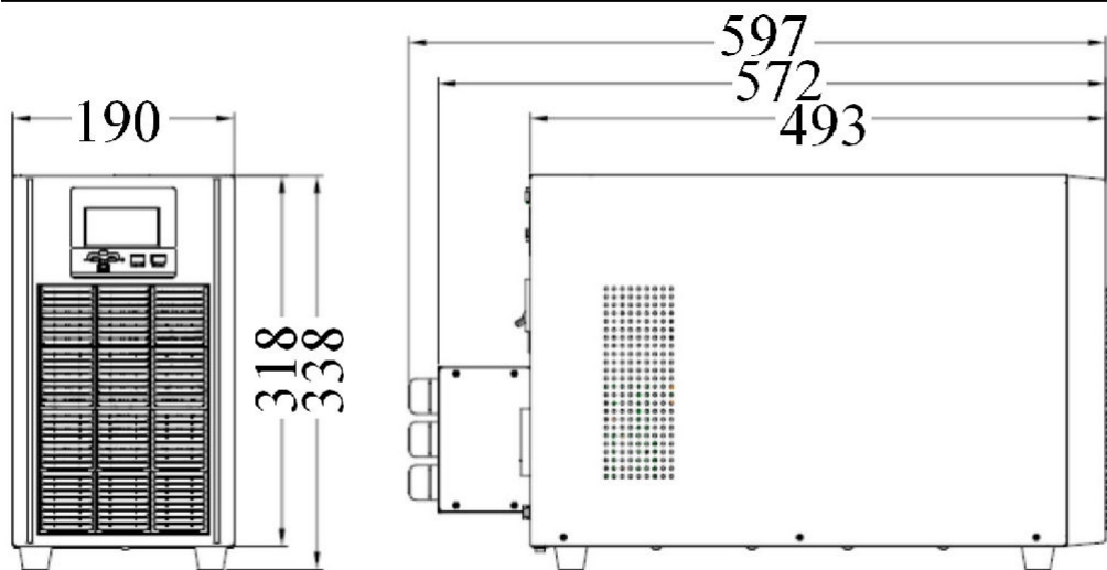
3. Modelos 10 e 12kVA - Bateria externa (Long)
