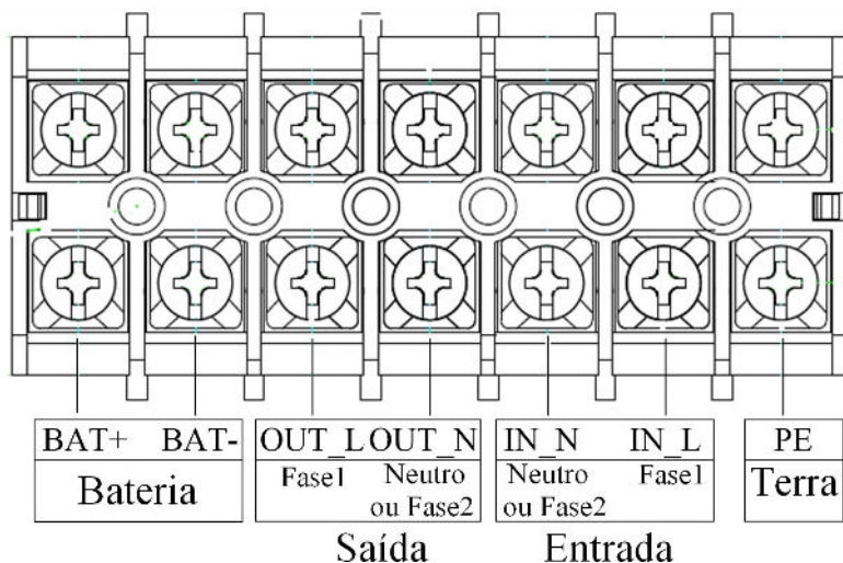
Fig 2- 1: Diagrama de fiação do bloco de terminais
